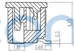
截面 A-A
