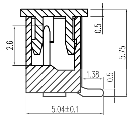
截面 A-A
