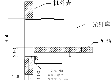
机外壳开口示意图
