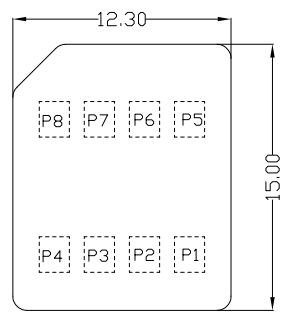
MICRO. SIM CARD
