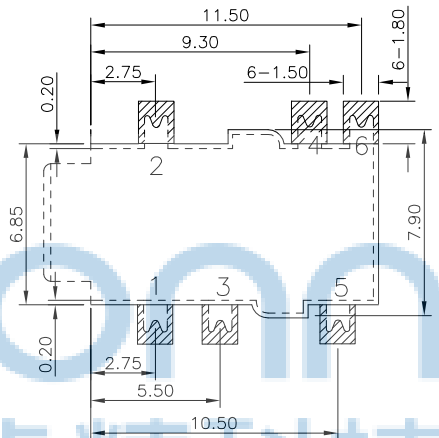
正贴 P.C.B LAYOUT TOP VIEW
