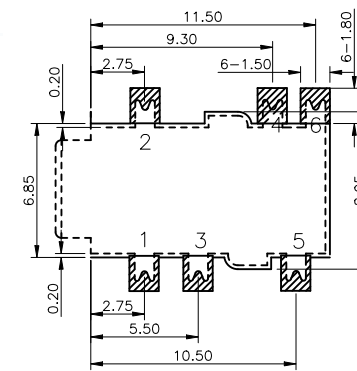
正贴 P.C.B LAYOUT TOP VIEW
