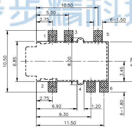
P.C.B LAYOUT TOP VIEW 反贴
