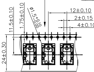
PJ25A001 载带图纸
