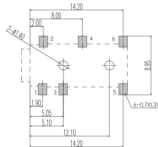
P.C.B LAYOU TOP VIEW
