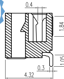
截面 A-A
