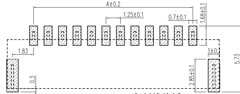
印制线路板
