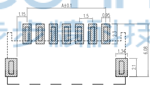
印制线路板
