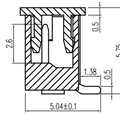
截面 A-A
