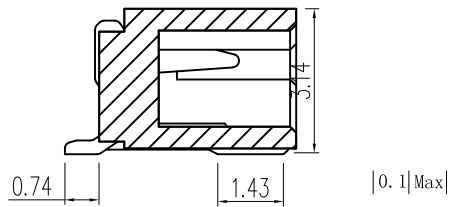
截面 A-A
