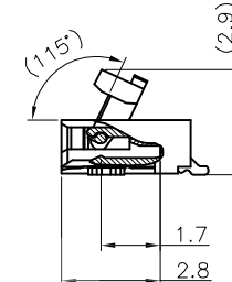
SECTION A-A SCALE 1:1
