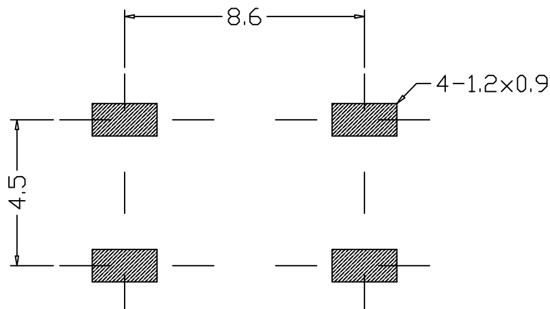
PCB线路板图
