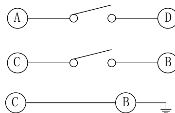
电路图
