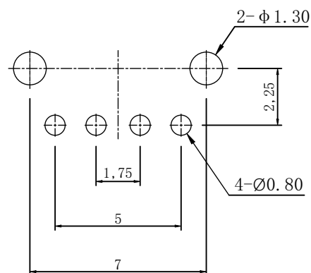
PCB. 焊接图
