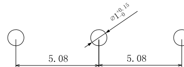
印制线路板 Recommended P.C.B layout
