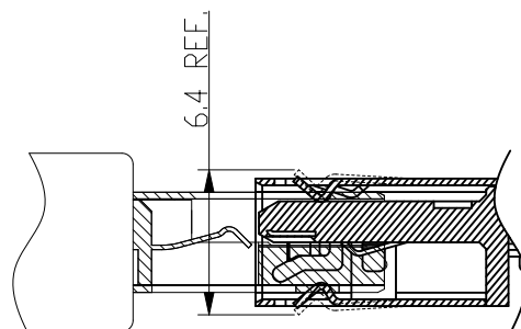
公母對插圖
