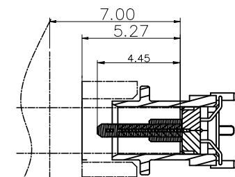
plug插入深度参考图
