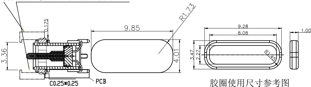
组装示意图
