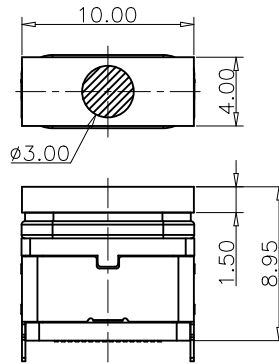
装前塞示意图
