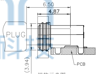
组装示意图
