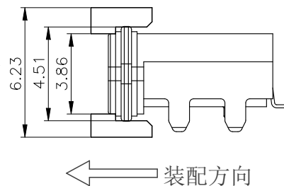
组装示意图
