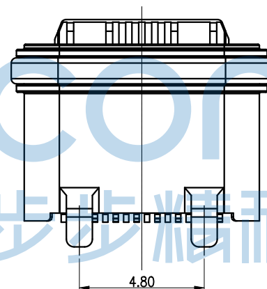
装前塞示意图
