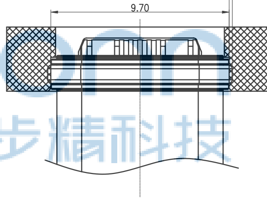
U型结构密封参考尺寸
