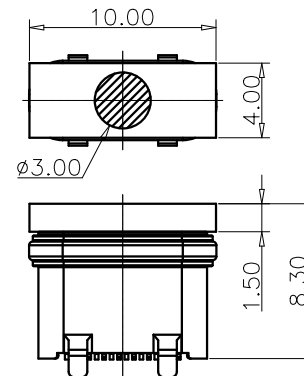
装前塞示意图
