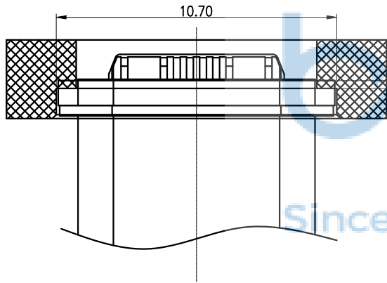
直压结构密封参考尺寸
