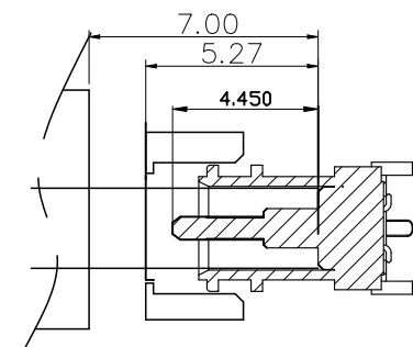
plug插入深度参考图
