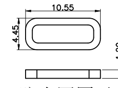
防水圈图示
