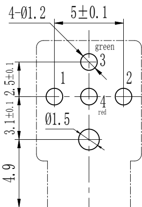
元件面孔位图
