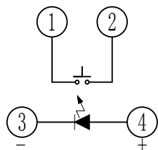
电原理图
