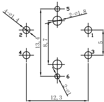
安装尺寸图
