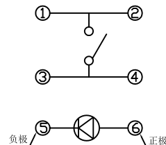
电路图
