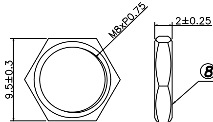
Nut
