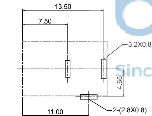
P. C. B 设计参考尺寸
