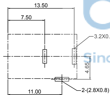
P.C.B 设计参考尺寸
