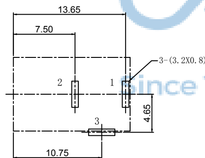
P.C.B 设计参考尺寸
