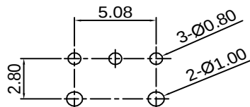
P.C.B 设计参考尺寸
