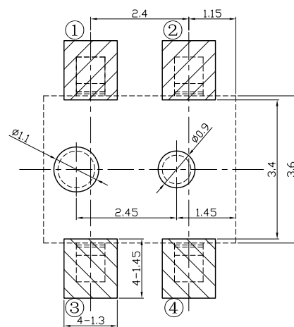
安装位置图
