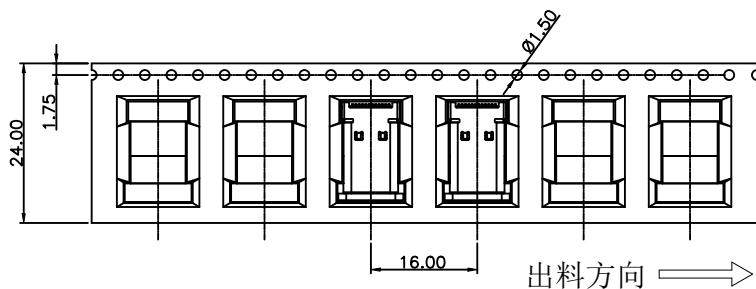
① 产品入载带示意图
