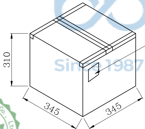
⑤ 外箱封箱示意图
