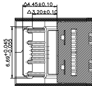
截面B-B
