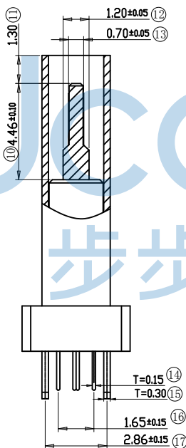
剖视图
