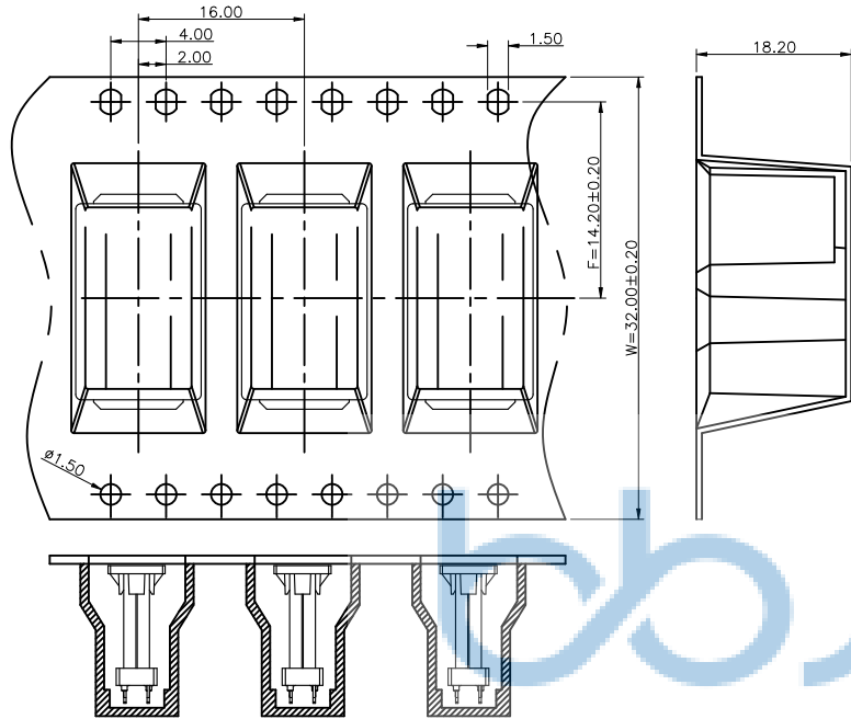
① 产品入载带示意图
