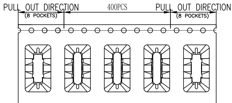
① 产品入载带示意图
