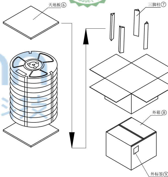
装箱示意图
