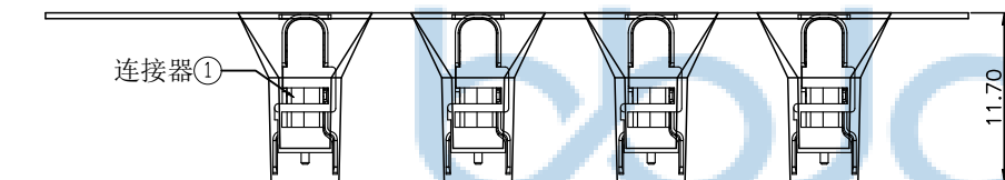
产品入载带示意图
