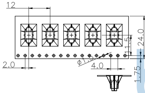
① 产品入载带示意图
