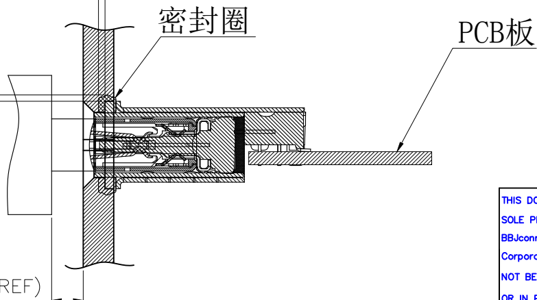
组装面板后公母头对插示意图
