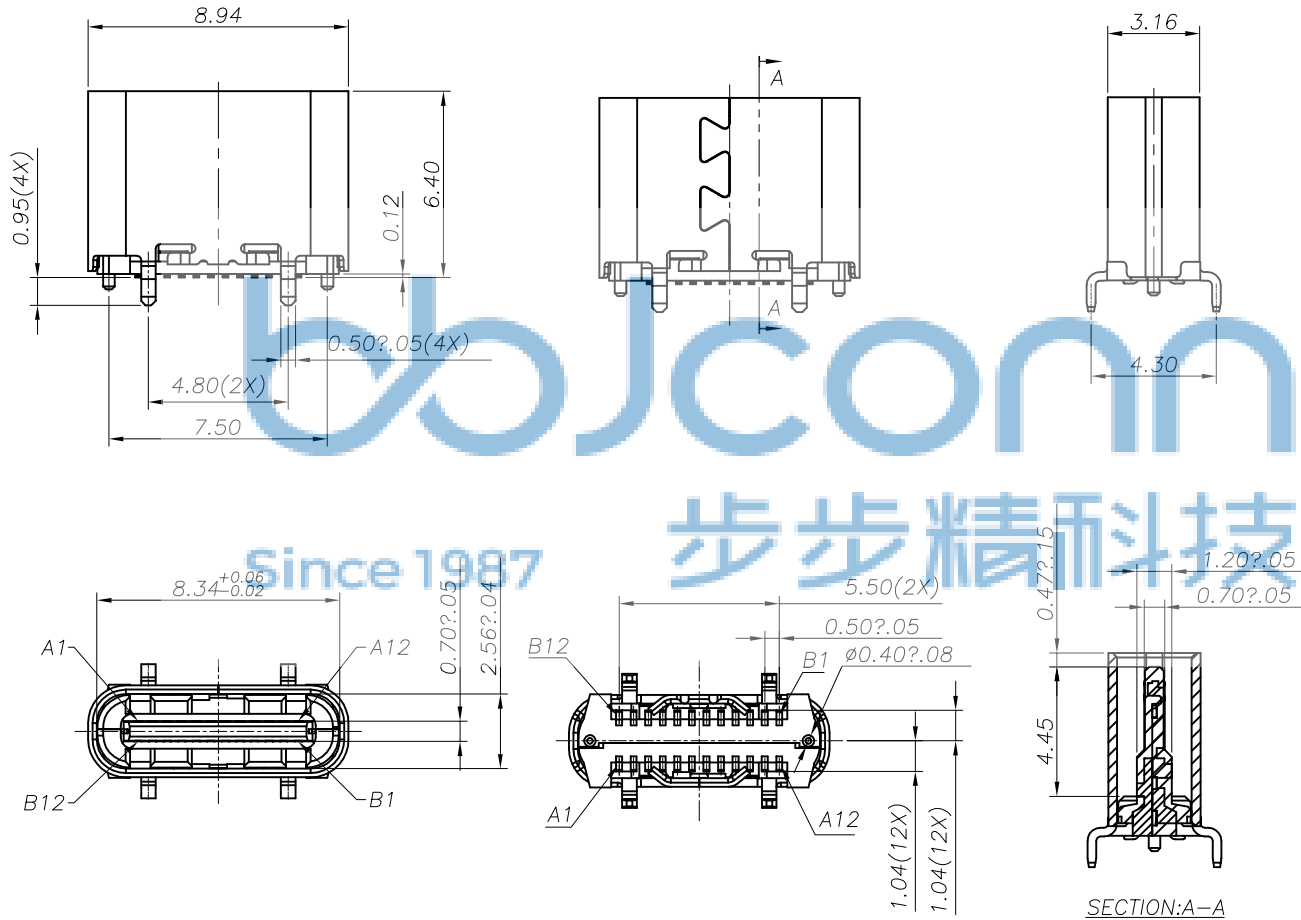
SECTION:A-A
