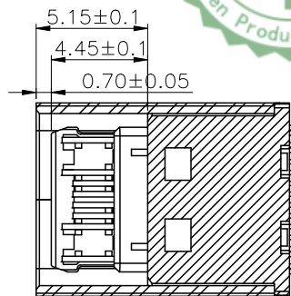
截面B-B
