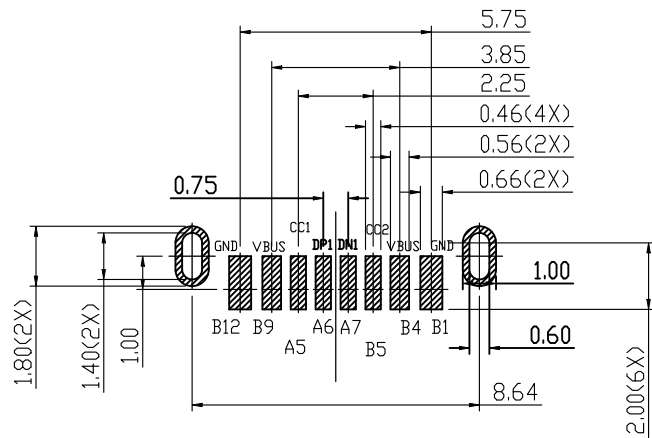
PCB参考图
