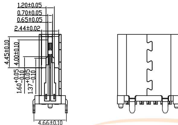
截面 1-1
