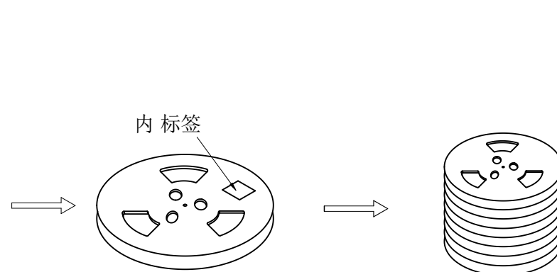
② 卷盘贴标签示意图
