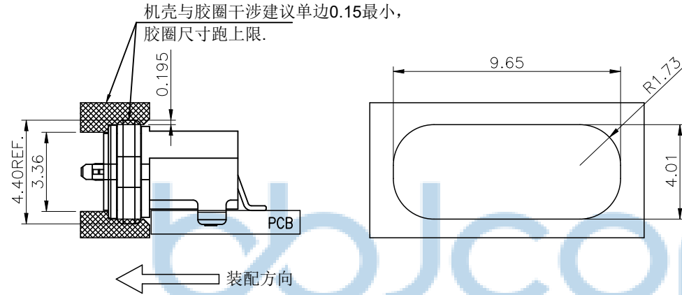
组装示意图
