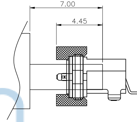
plug插入深度参考图
